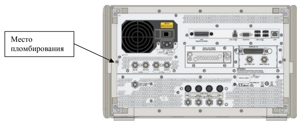
Рисунок 2 - Внешний вид анализаторов E5080A, вид сзади (схематично)
